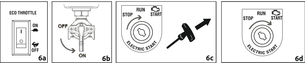
Рисунок 6 – Ручной и электрический запуск
