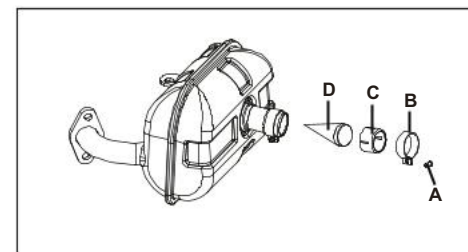
Рисунок 12 – Очистка искрогасителя
