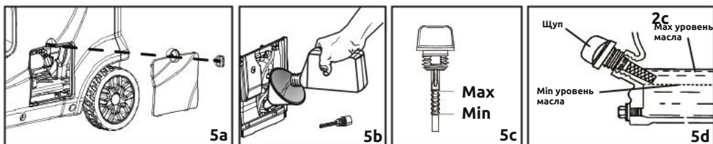
Рисунок 5 - Уровень масла
