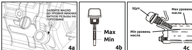
Рисунок 4 - Уровень масла
