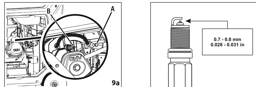
Рисунок 9 – Установка свечи
