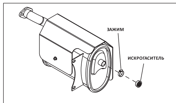
Рисунок 9 – Искрогаситель
