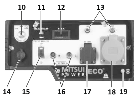
ПАНЕЛЬ УПРАВЛЕНИЯ ZM 10000 EA
