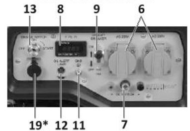
ПАНЕЛЬ УПРАВЛЕНИЯ ZM 7500 EA
