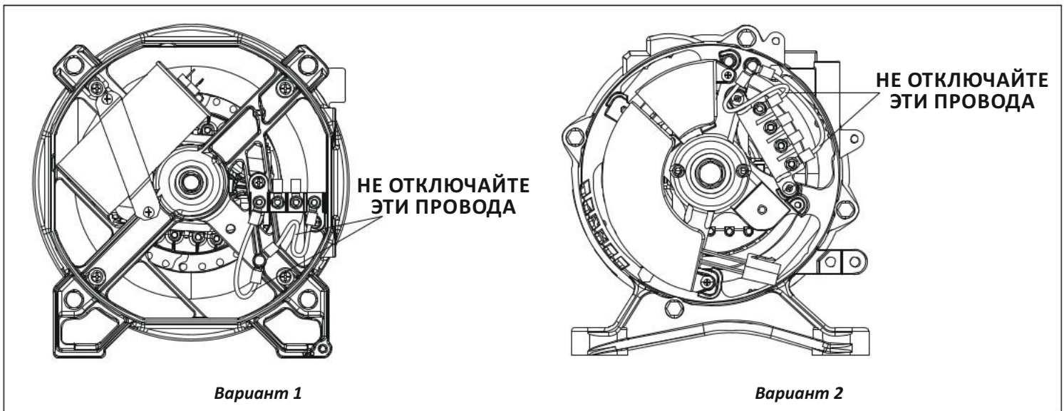
Рисунок 4 - Заземление нейтрали
