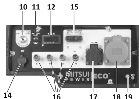
ПАНЕЛЬ УПРАВЛЕНИЯ ZM 10000 EA-3
