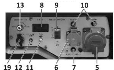
ПАНЕЛЬ УПРАВЛЕНИЯ ZM 6500 E, ZM 8500 E
