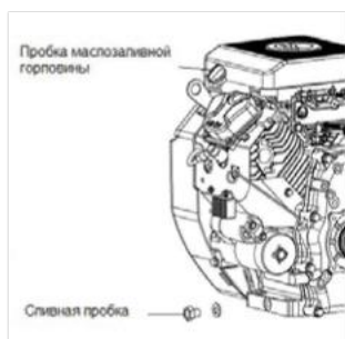
Рисунок 3. Проверка уровня моторного масла.
