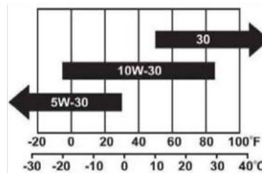
Рисунок 5. Зависимость класса вязкости моторного масла от температуры окружающей среды.
