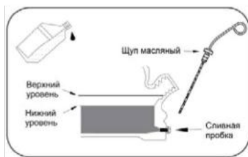
Рисунок 4. Отметки на масляном щупе.
