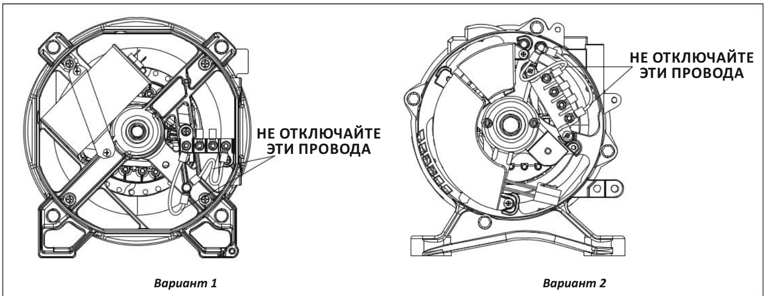
Рисунок 4 - Заземление нейтрали
