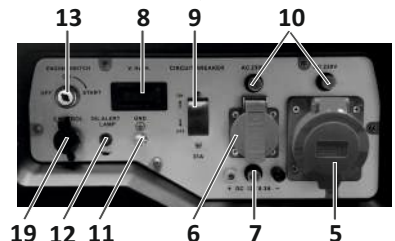
ПАНЕЛЬ УПРАВЛЕНИЯ ZM 6500 E, ZM 8500 E, ZM 9500 E, ZM 9500 E-3
