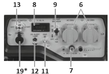
ПАНЕЛЬ УПРАВЛЕНИЯ ZM 7500 EA, ZM 9500 EA
