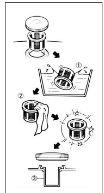
Рисунок 15 – Очистка фильтра топливного бака
