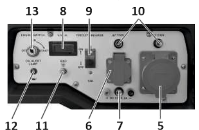
ПАНЕЛЬ УПРАВЛЕНИЯ ZM 6500 E, ZM 8500 E, ZM 9500 E, ZM 9500 E-3
