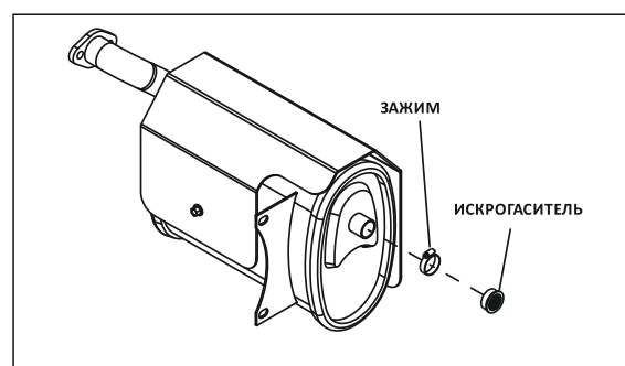
Рисунок 9 – Искрогаситель
