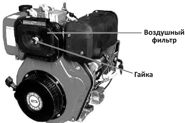
Рисунок 6 – Очистка воздушного фильтра
