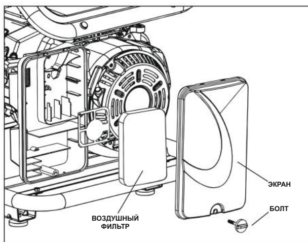
Рисунок 8 – Воздушный фильтр
